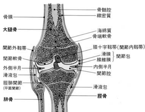
図① 関節の構造（膝を横から見た図）
